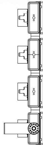
左视图
