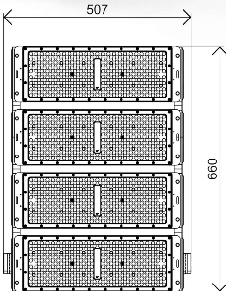
主视图
